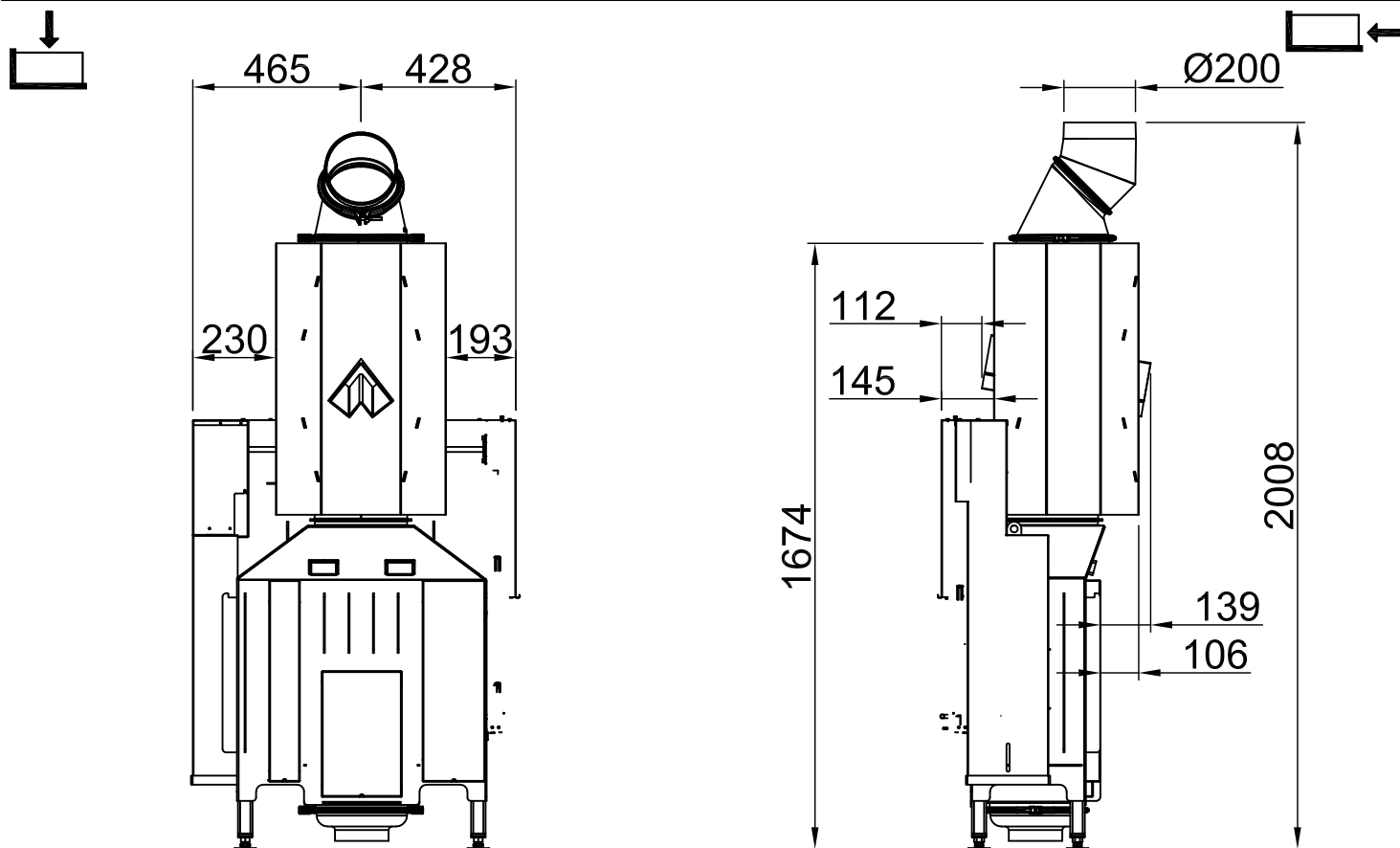
~1:20 Thermobox, wąski
