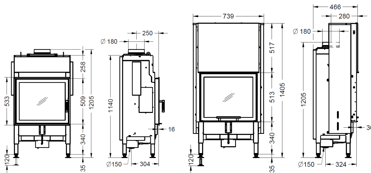
Global 1Vh 60
