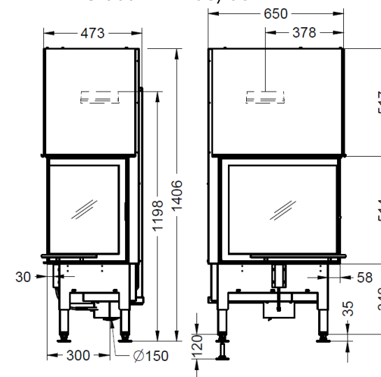
Global 2Rh 58/39
