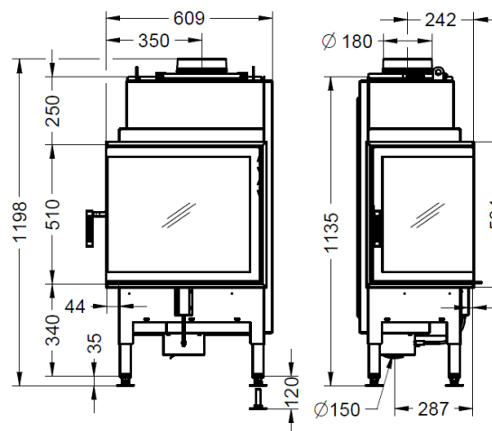
Global 2L 39/58
